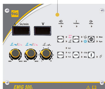
ПАНЕЛЬ УПРАВЛЕНИЯ
